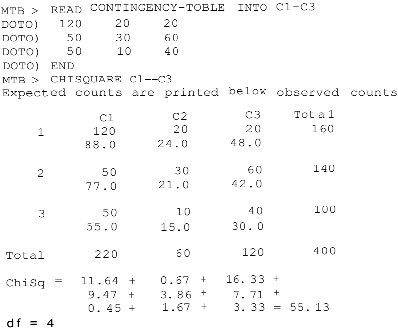
Fig. 12-1 Listado de Minitab
